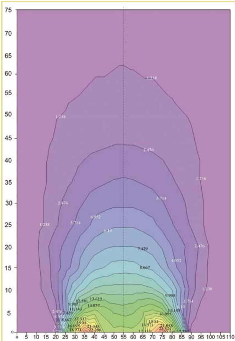
Распространенность магнитного поля от индуктора аппарата «АЛМАГ-01»; по вертикали – глубина проникновение магнитного поля, в мм; по горизонтали – распространенность магнитного поля от центра индуктора, в мм; по силовым линиям – напряженность магнитного поля на различной глубине в милитеслах (мТл)
